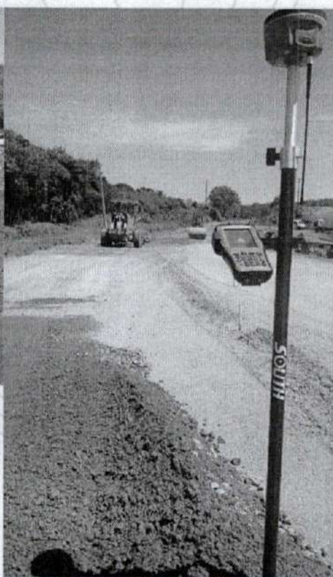
Locação Topográfica e acompanhamento de Obra de uma ponte sobre o Rio Andrada, situada em Boa Vista da Aparecida.
